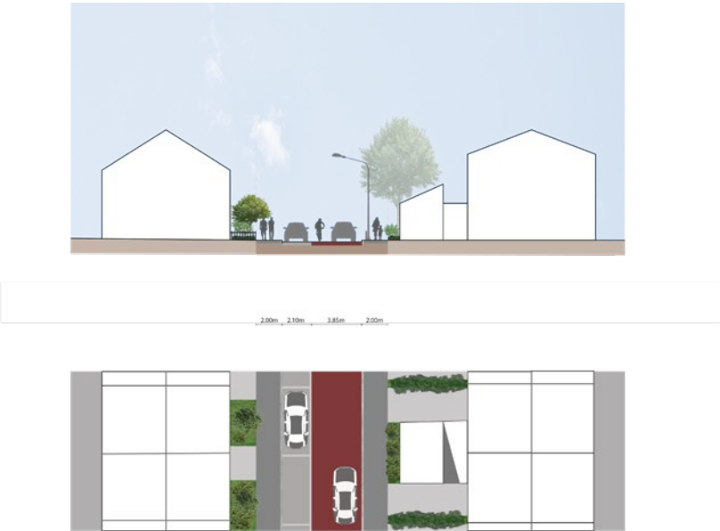
Profiel woonstraat 9.95m huidige situatie
